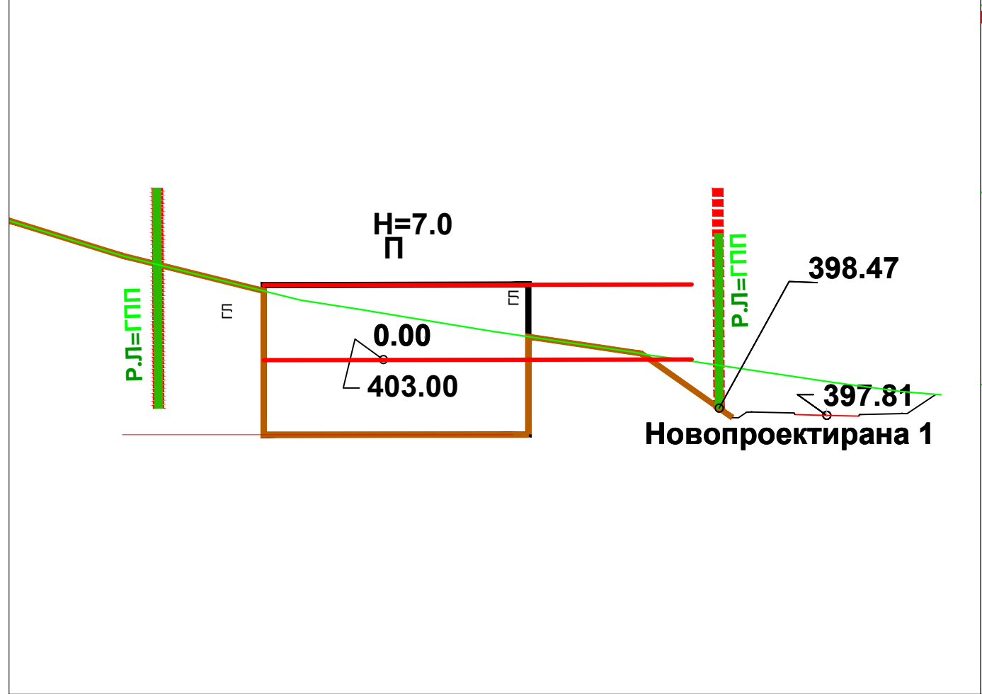
ПРЕСЕК А-А
